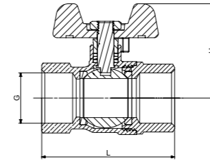
PİRİNÇ VANALAR PN25 Kelebek Saplı Kresel Vana (Diřli)
