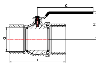
PİRİNÇ VANALAR PN16 Kresel Vana (Diřli, Ekonomik)
