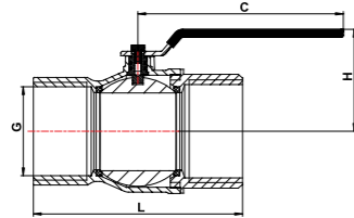
PİRİNÇ VANALAR PN10 İme Suyu Kresel Vana (Diřli, Uzun)
